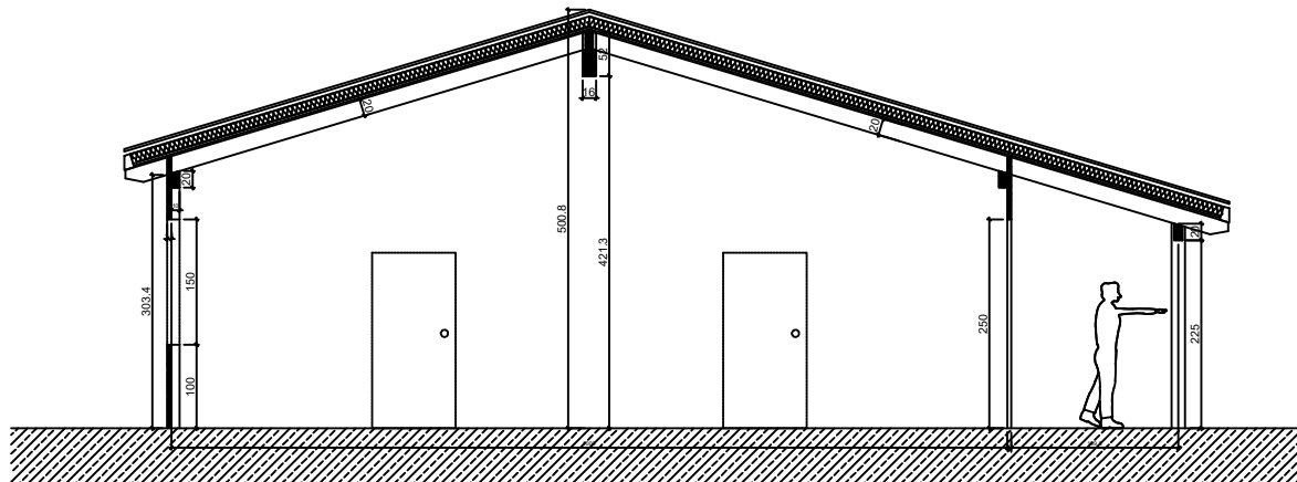
SEZIONE AA
