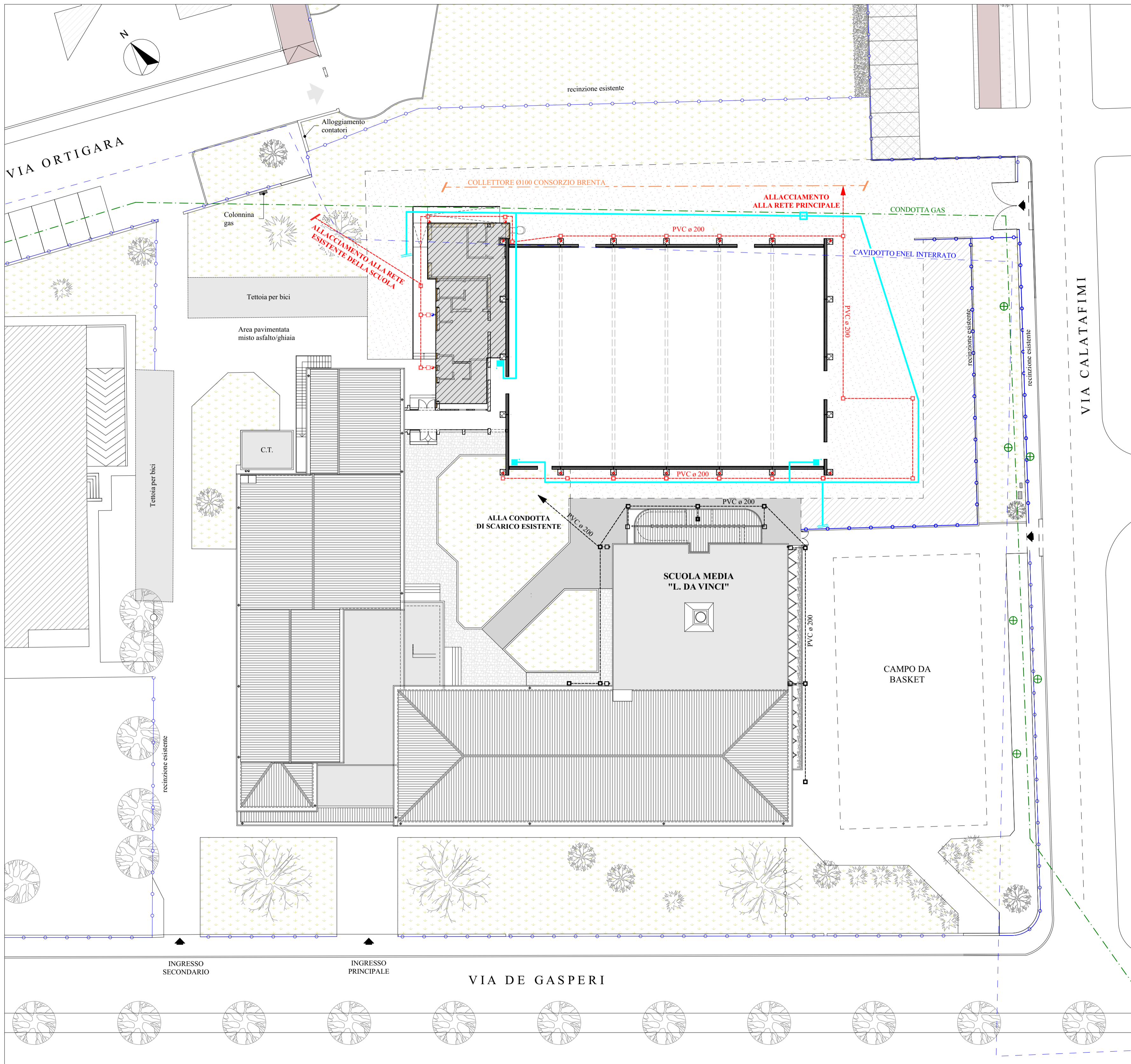
PLANIMETRIA RETE ACQUE BIANCHE
